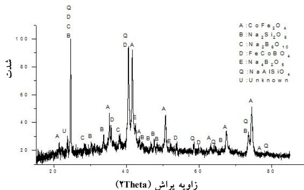
شکل ۷- الگوی XRD نمونه عملیات حرارتی شده در دمای 670 درجه سانتی‌گراد به مدت یک ساعت
