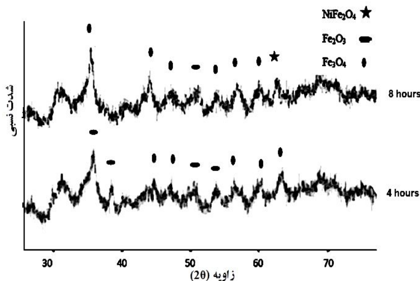
شکل ۱- الگوهای پراش پرتو اشعه ایکس نمونه‌های تولید شده در 180^\circ درجه سانتی‌گراد در زمان‌های ۴ و ۸ ساعت
