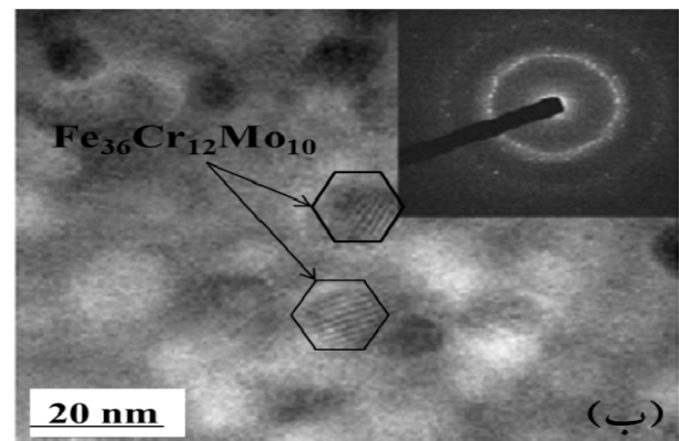
شکل ۸- ساختار میکروسکوپ الکترونی عبوری آلیاژ \text{Fe}_{51}\text{Cr}_{18}\text{Mo}_7\text{B}_{16}\text{C}_4\text{Nb}_4 در حالت: (الف) غیربلورین و (ب) تبلور یافته
