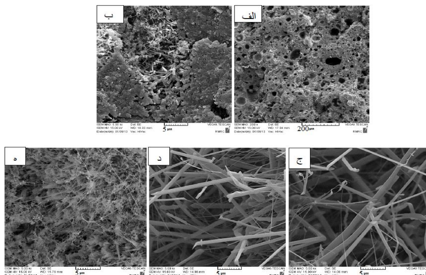
شکل ۵- تصاویر میکروسکوپ الکترونی رویشی SEM از نمونه‌های: (الف) B1، (ب) B2، (ج) B4، (د) B5 و (ه) B6 که برحسب افزایش مقدار کلرید آمونیوم از صفر تا ۵۰ درصد وزنی می باشد
