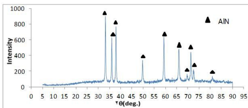
شکل ۷- الگوی پراش اشعه X (XRD) از نمونه حاوی پودر آلومینیوم با اندازه ذرات ۴۵ میکرومتر و ۵۰٪ وزنی کلرید آمونیوم
