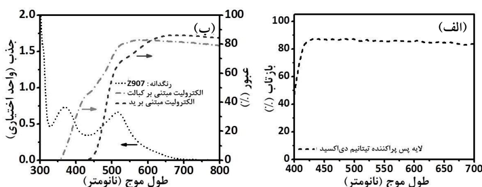
شکل ۳- (الف) طیف بازتاب پخش‌ی لایه پس‌پراکنده تیتانیم دی‌اکسید و (ب) طیف جذب رنگدانه Z907 که از سطح الکتروود نوری در دی‌متیل‌فرامید واجذب شده است (نقطه‌چین) و طیف عبور الکتروولیت Z959 (مبتنی بر ید) (خط‌چین) و Z1147 (مبتنی بر کبالت) (نقطه-خط‌چین)
