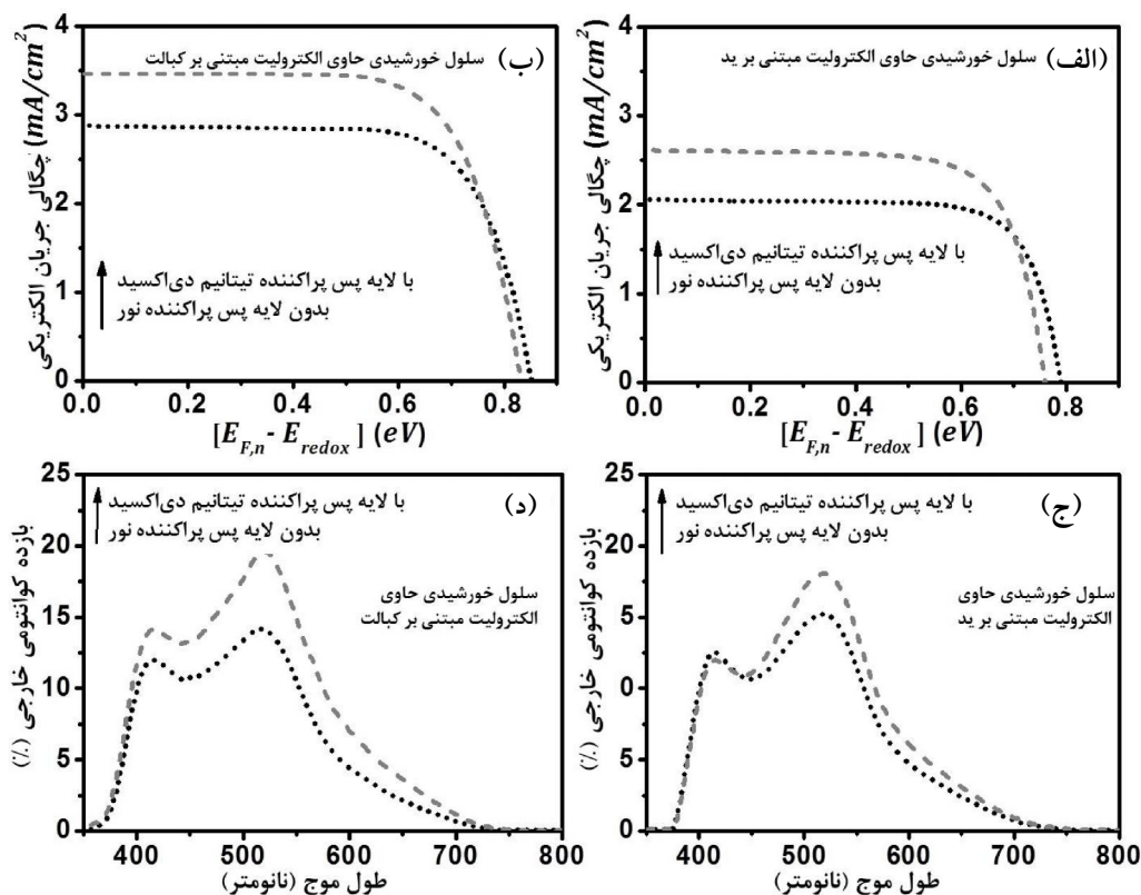
شکل ۴- منحنی چگالی جریان - ولتاژ سلول‌های خورشیدی رنگدانه‌ای: (الف) حاوی الکترولیت مبتنی بر ید، (ب) حاوی الکترولیت مبتنی بر کبالت. منحنی بازده کوانتومی خارجی سلول‌های خورشیدی، (ج) حاوی الکترولیت مبتنی بر ید و (د) حاوی الکترولیت مبتنی بر کبالت. (نقطه چین: سلول خورشیدی رنگدانه‌ای مرجع بدون به کارگیری لایه پس پراکننده نور، خط چین: سلول خورشیدی اصلاح شده با پس پراکننده تیتانیم دی اکسید)
