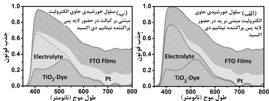
شکل ۶- جذب فوتون در سلول‌های حاوی الف) الکترولیت مبتنی بر ید و ب) الکترولیت مبتنی بر کبالت در حضور لایه پس پراکنده‌ی نور که نشان می‌دهند در هر طول موج چه درصدی از فوتون فرودی به وسیله‌ی شیشه FTO یا لایه‌ی تیتانیم دی اکسید حساس شده به رنگدانه یا الکترولیت و یا پلاتین جذب می‌شود.
