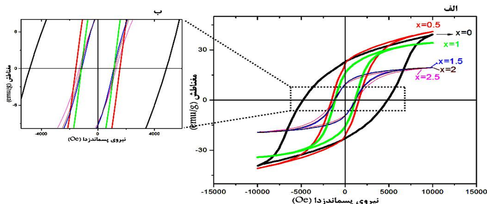
شکل ۹- الف) حلقه‌های پسماند نانو ذرات فریت استرانسیم با ترکیب \text{SrFe}_{12-2x}(\text{MgCo})_{0.5x}\text{Ti}_x\text{O}_{19} به ازا x=0-2.5 ، ساخته شده در دمای 900^\circ\text{C} به مدت ۱ ساعت و ب) نمایش تغییرات نیروی پسماندزدا در بزرگ‌نمایی بیشتر
