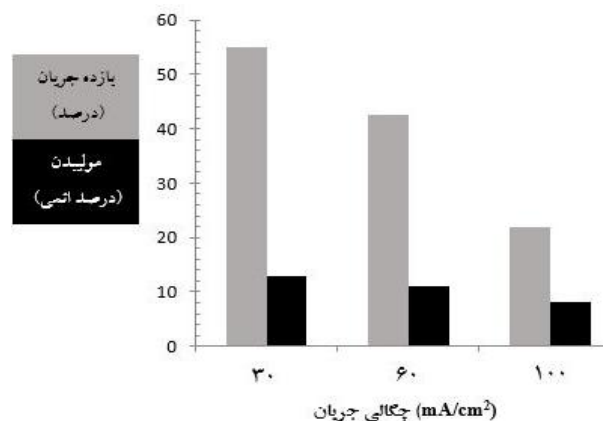
شکل ۳- بازده حمام و درصد اتمی مولیبدن پوشش برحسب چگالی جریان پوشش‌دهی
