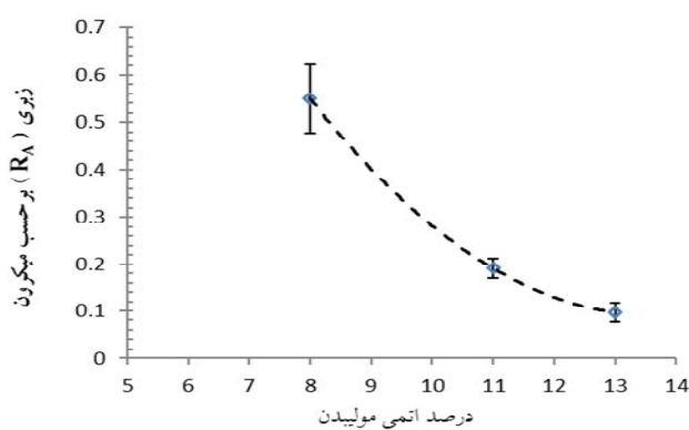
شکل ۶ - زبری پوشش‌های رسوب الکتریکی Ni-Mo بر حسب مقدار مولیبدن پوشش
