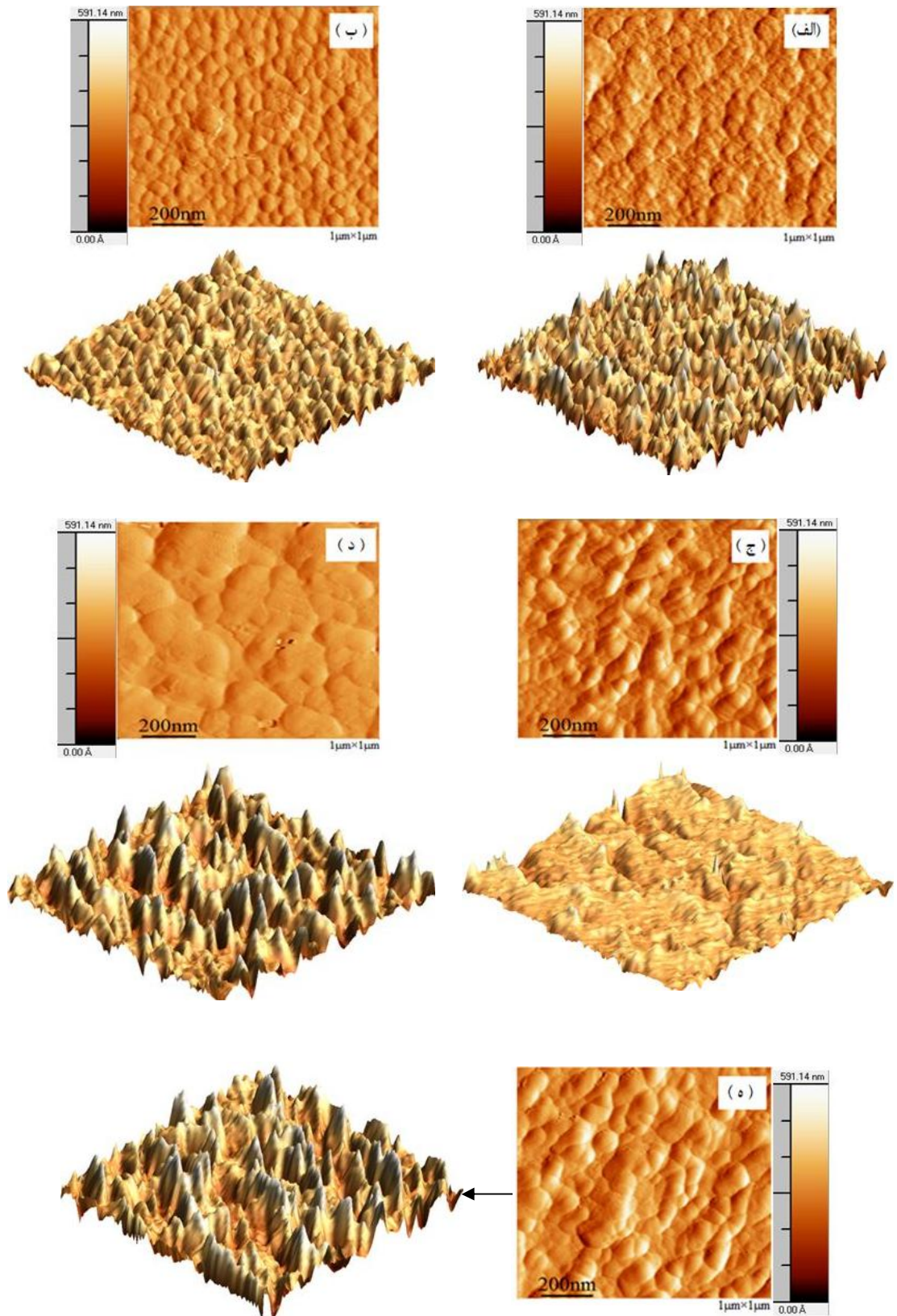
شکل ۴- تصاویر میکروسکوپی روبشی لایه‌های نازک نئودمیوم آهن بور در دمای آنیل مختلف: الف) (۴۵°، ب) (۵۰°، ج) (۵۵°، د) (۶۰° و ه) (۶۵° درجه سانتی‌گراد
