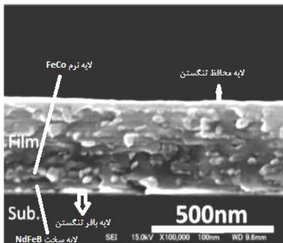
شکل ۴- سطح مقطع لایه چندگانه [NdFeB(20nm)/FeCo(20nm)] \times 9
