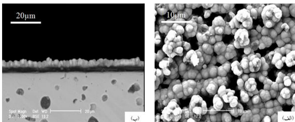
شکل ۸- تصویر میکروسکوپی الکترونی روبشی از نمونه پوشش داده شده با چگالی جریان 250 میلی آمپر بر سانتی متر مربع به مدت 20 دقیقه: (الف) سطح پوشش و (ب) سطح مقطع پوشش
