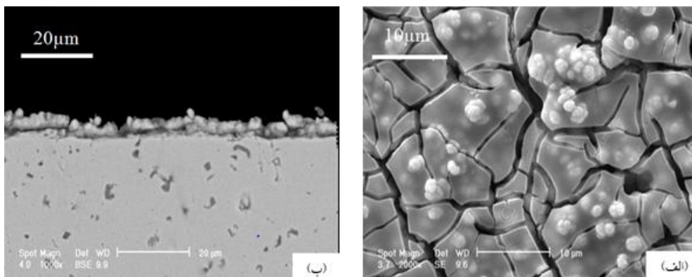
شکل ۷- تصویر میکروسکوپی الکترونی روبشی از نمونه پوشش داده شده با چگالی جریان 200 میلی آمپر بر سانتی متر مربع به مدت 20 دقیقه: (الف) سطح پوشش و (ب) سطح مقطع پوشش
