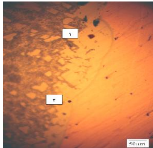
شکل ۹- اثرات فرورونده‌های هرمی در آزمون ریزسختی سنجی در نمونه A800C25. نقطه ۱ واقع در منطقه فاز ۲ و نقطه ۲ واقع در منطقه است.
