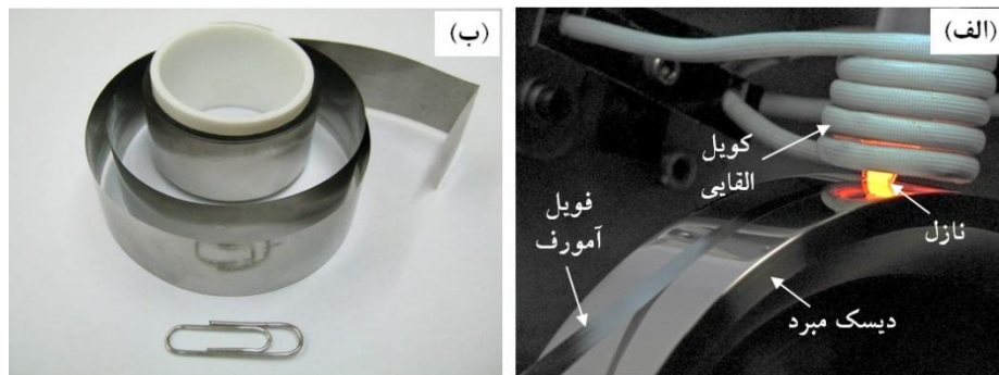
شکل ۱- الف) فرایند ریخته ریزی نوارهای عریض و ب) نمونه‌ای از فویل آمورف MBF-20 تولیدی
