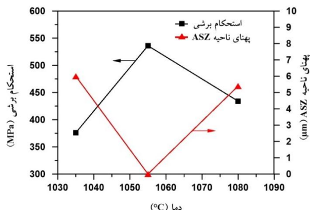
شکل ۱۴- تغییرات استحکام برشی و ضخامت ناحیه ASZ نمونه‌های اتصال داده شده در دماهای مختلف و زمان 30 دقیقه با استفاده از فولیل آمورف تک لایه
