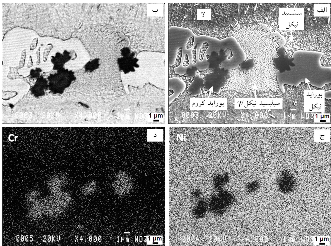
شکل ۷- تصاویر SEM از ناحیه اتصال TLP در دمای ۱۰۸۰ درجه سانتی گراد به مدت ۳۰ دقیقه با استفاده دولایه فویل آمورف، (الف) الکترون‌های ثانویه، (ب) الکترون‌های برگشتی، (ج) و (د) به ترتیب آنالیز نقشه اشعه ایکس عناصر نیکل و کروم
