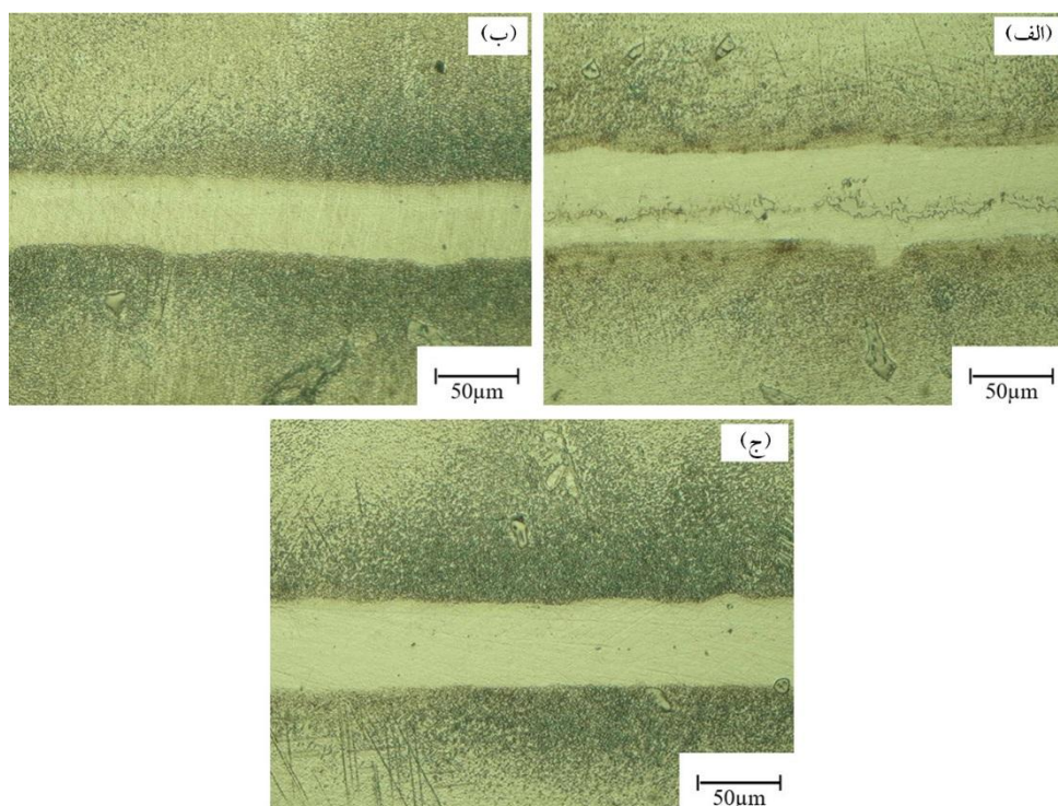
شکل ۱۱- (رنگی در نسخه الکترونیکی) تصاویر میکروسکوپی نوری از ریزساختار ناحیه اتصال ایجاد شده به وسیله یک لایه فویل آمورف در دمای ۱ درجه سانتی گراد ۸۰° و زمان های، الف) ۳۰، ب) ۴۵ و ج) ۶۰ دقیقه
