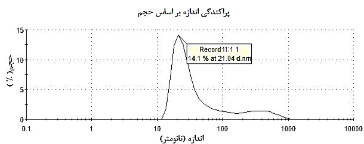
شکل ۶- نمودار توزیع اندازه ذرات توسط آزمون پراکندگی دینامیکی نور مربوط به نمونه بهینه
