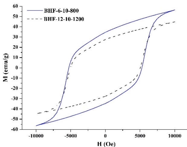
شکل ۶- حلقه پسماند نمونه هگزارفیت باریم سنتز شده با نسبت‌های مولی آهن/باریم برابر با ۱۲ و ۶
