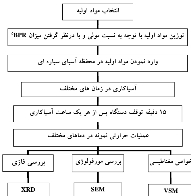
شکل ۱- روند نمای تهیه هگزاferit باریم به روش فعال‌سازی مکانیکی
