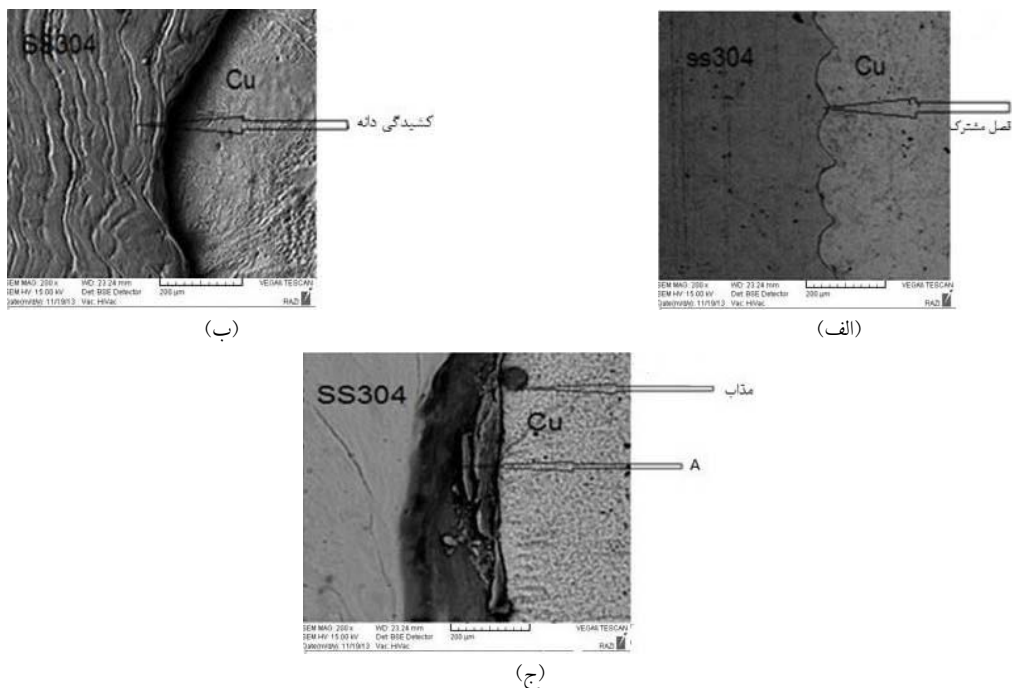
شکل ۶- تصاویر میکروسکوپی الکترونی روبشی فصل مشترک، آزمون یک: الف) فصل مشترک ب) کشیدگی دانه و ج) منطقه ذوب موضعی A
