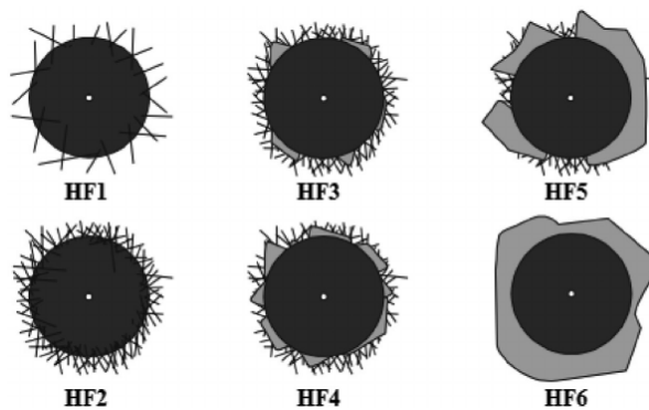
شکل ۱- کلاس بندی چسبندگی پوشش در استاندارد VDI 3198 [۱۴]
