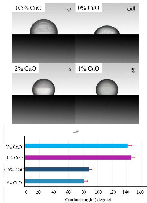
شکل ۴- تصاویر مربوط به شکل قطره آب بر سطح پوشش پلی‌دی‌متیل‌سیلوکسان- اکسید سیلیسیم و با مقادیر مختلفی از اکسید مس (الف) صفر، (ب) ۰/۵، (ج) ۱، (د) ۲ درصد وزنی و (ه) نمودار ستونی میانگین زاویه ترشوندگی نمونه‌ها (رنگی در نسخه الکترونیکی)
