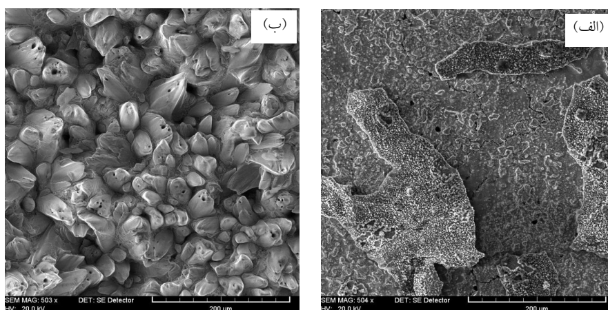
شکل ۸- تصاویر میکروسکوپی الکترونی روبشی مورفولوژی سطح نمونه: (الف) بدون پوشش و (ب) و نمونه پوشش داده شده بعد از اکسیداسیون سیکلی در دمای ۱۰۰۰ درجه سانتی‌گراد
