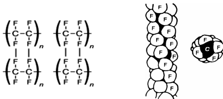
شکل ۸- نحوه قرارگیری اتم‌ها در پلی تترا فلئوراتیلن [۲۹]
