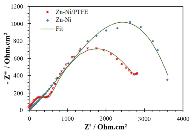
شکل ۶- نمودار نایکوئیست پوشش Zn-Ni و Zn-Ni/PTFE در محلول ۳/۵ wt.% NaCl
