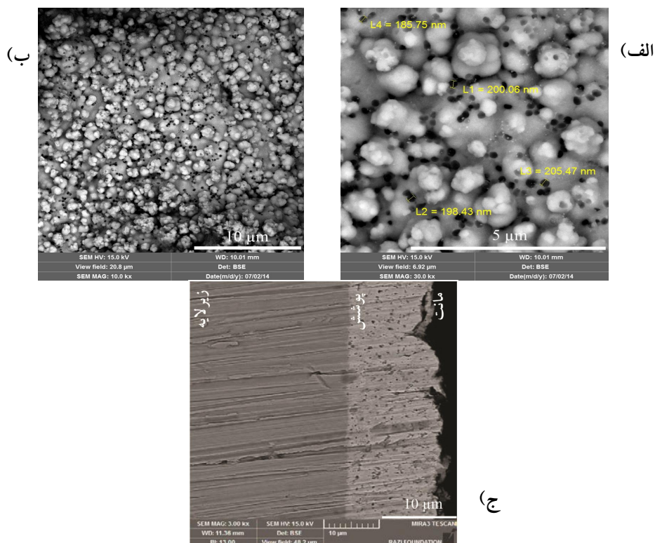
شکل ۱- تصاویر میکروسکوپ الکترونی روبشی با بزرگنمایی مختلف از توزیع مناسب ذرات در پوشش کامپوزیتی Zn-Ni/PTFE با غلظت سه گرم بر لیتر ذرات پلی تترا فلوئوراتیلن: الف و ب) سطح پوشش و ج) مقطع پوشش
