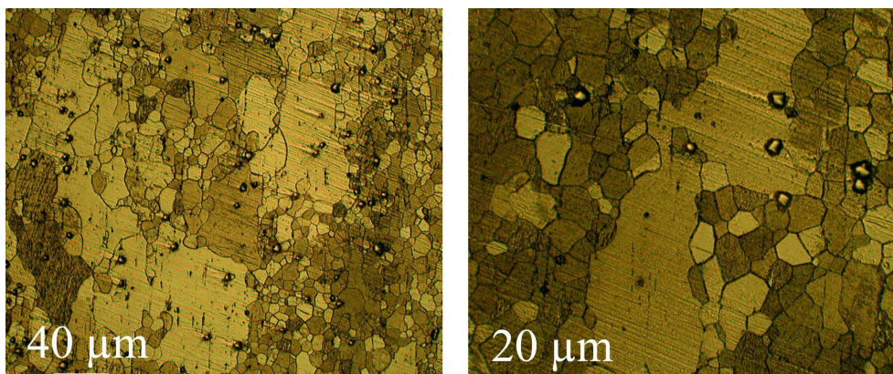
شکل ۸- تصاویر میکروسکوپی نوری نشان‌دهنده رشد دانه‌های غیریکنواخت در آلیاژ Mg-۳Gd-۳Al-Zn در دو بزرگنمایی متفاوت
