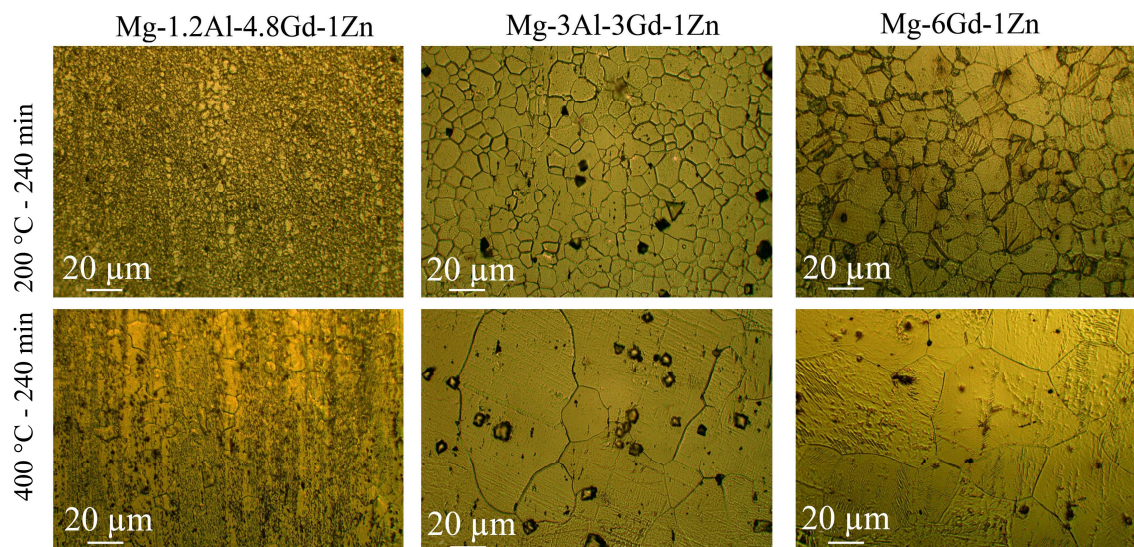
شکل ۲- تصاویر میکروسکوپی نوری در حالت آنیل در دما و زمان‌های مختلف
