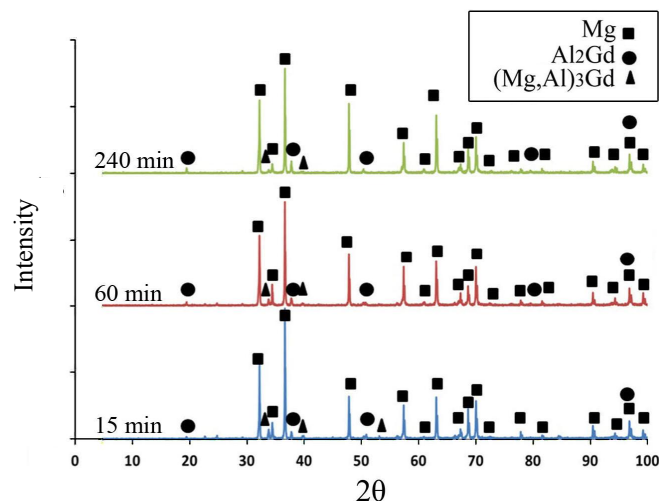
شکل ۳- الگوی پراش پرتو ایکس آلیاژ \text{Mg-4.8\%Gd-1.2\%Al-1\%Zn} آنیل شده در دمای 500^\circ\text{C} در زمان‌های مختلف
