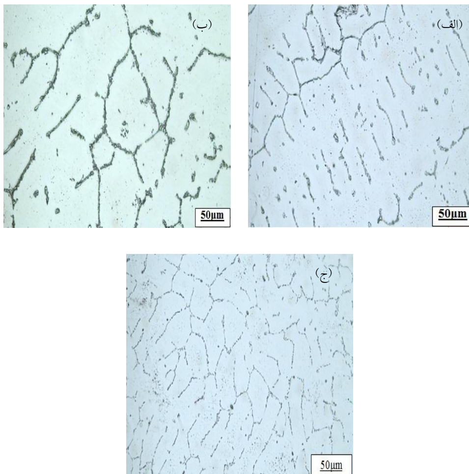
شکل ۲- تصاویر متالوگرافی آلیاژهای: الف) \text{Fe}_3\text{Al-0.5B} ، ب) \text{Fe}_3\text{Al-0.5Zr} و ج) \text{Fe}_3\text{Al-0.5Zr0.5B}
