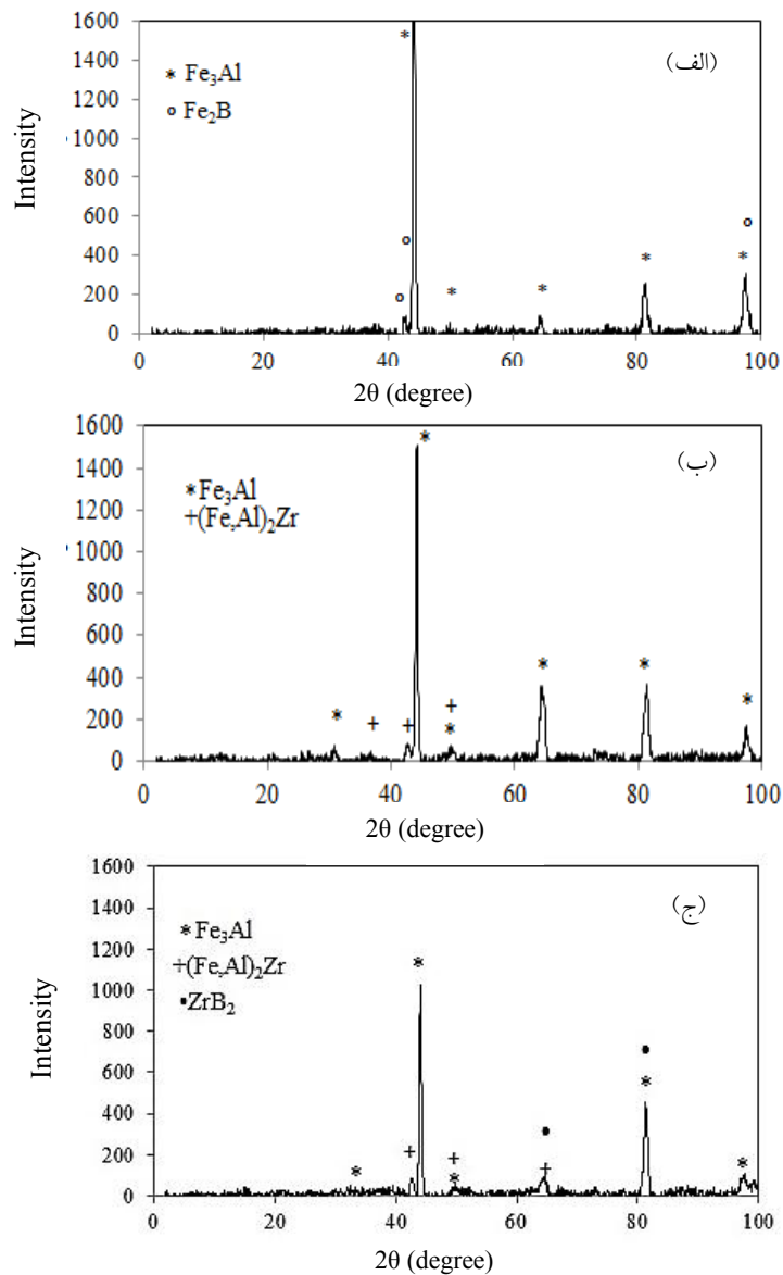
شکل ۵- الگوی پراش پرتو ایکس برای آلیاژهای: الف) \text{Fe}_3\text{Al} -۰.۵B، ب) \text{Fe}_3\text{Al} -۰.۵Zr و ج) \text{Fe}_3\text{Al} -۰.۵Zr۰.۵B
