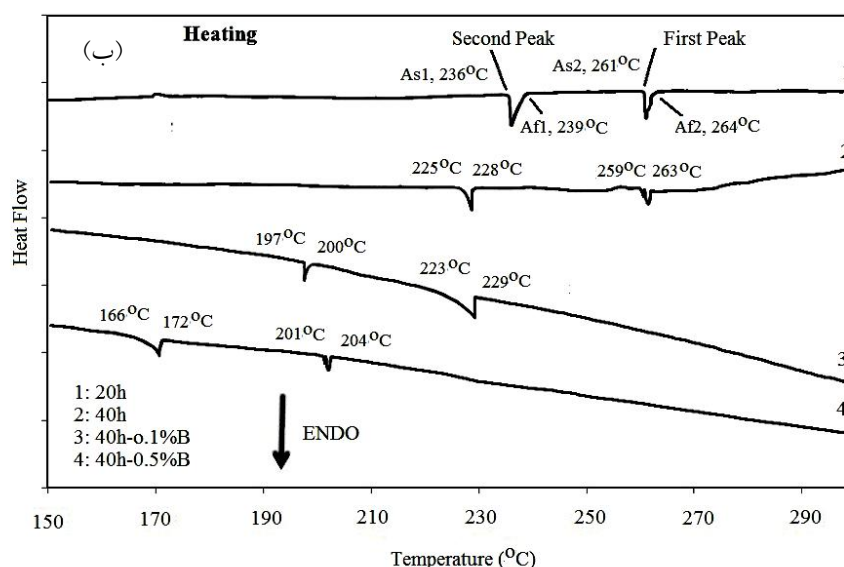
شکل ۷- نمودارهای آزمون گرماسنجی تفاضلی روشی مربوط به سیکل‌های سرمایش و گرمایش نمونه‌های ۲۰ و ۴۰ ساعت آسیاکاری شده و ۴۰ ساعت آسیاکاری شده حاوی ۰/۱ و ۰/۵ درصد بور
