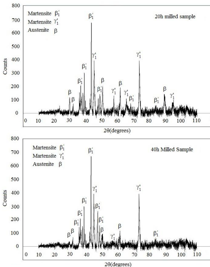
شکل ۱- الگوی پراش پرتو ایکس نمونه های ۲۰ و ۴۰ ساعت آسیاکاری شده پس از عملیات حرارتی حل سازی و کوئنچ.
