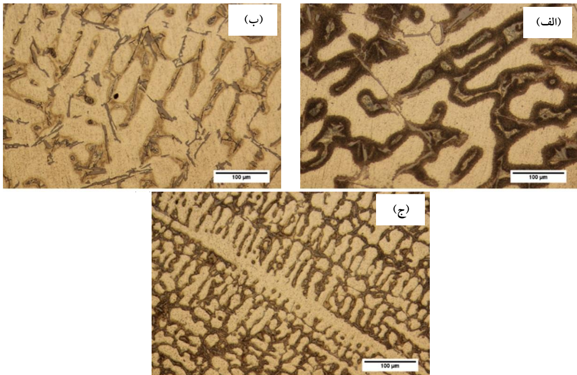
شکل ۲- تیغه‌های سیلیسیم یوتکتیکی آلیاژ AS7U3G در بزرگنمایی بالا: الف) قالب ماسه‌ای، ب) قالب فلزی پیش‌گرم شده و ج) قالب فلزی آب‌گرم
