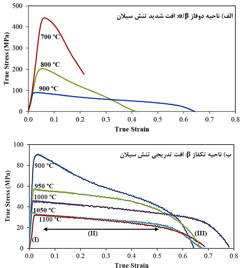
شکل ۳- نمودار تنش - کرنش حقیقی حاصل از آزمایش کشش گرم شمش ریختگی آلیاژ SP-700 در دماهای ۷۰۰-۱۱۰۰ درجه سانتی گراد با نرخ کرنش ۱/۰ بر ثانیه: الف) محدوده دمایی دوفاز و ب) محدوده دمایی تکفاز
