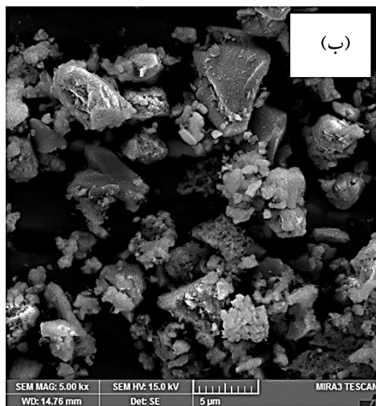
شکل ۱- تصاویر میکروسکوپی الکترونی روبشی الکترون ثانویه از مورفولوژی ذرات: الف) زیرکونیم و ب) تیتانیوم
