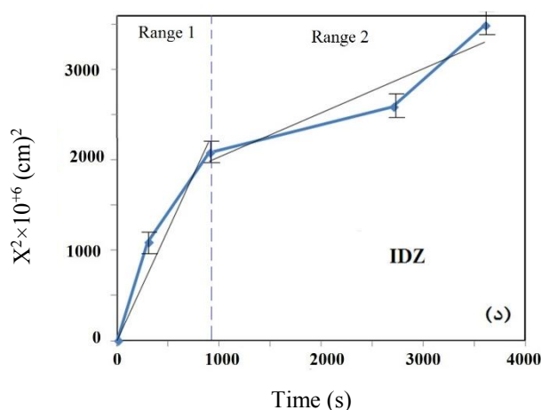
شکل ۵- الف و ب) تغییرات ضخامت پوشش بورایدی و لایه تحت نفوذ در زمان‌های مختلف، ج و د) برازش مدل سینتیکی بر تغییرات مربع عمق نفوذ ( X^2 ) بر حسب زمان ( t )
