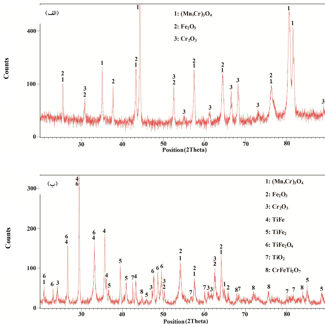
شکل ۶- الگوی پراش اشعه ایکس نمونه‌های: الف) بدون پوشش و ب) پوشش داده شده با تیتانیوم بعد از ۲۰۰ ساعت اکسیداسیون در دمای ۹۰۰ درجه سانتی‌گراد
