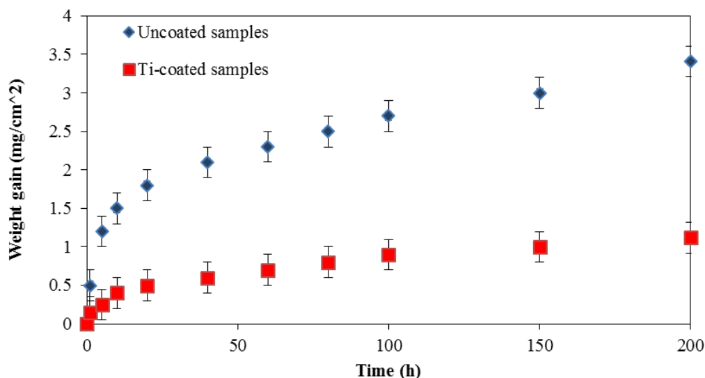
شکل ۴- افزایش وزن نمونه‌های بدون پوشش و نمونه‌های پوشش‌دار در طول اکسیداسیون هم‌دما
