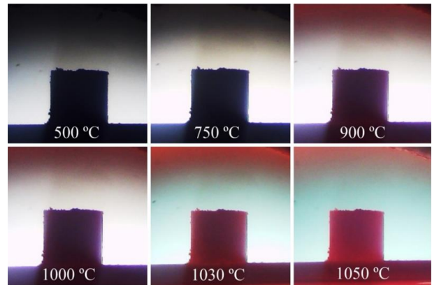
شکل ۱- تصاویر میکروسکوپی حرارتی از ترکیب سرپاره خالص (رنگی در نسخه الکترونیکی)
