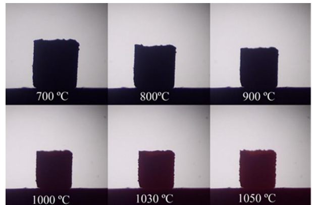
شکل ۳- تصاویر میکروسکوپی حرارتی از ترکیب کامپوزیت سرپاره و ۵۰ قسمت وزنی شیشه (رنگی در نسخه الکترونیکی)
