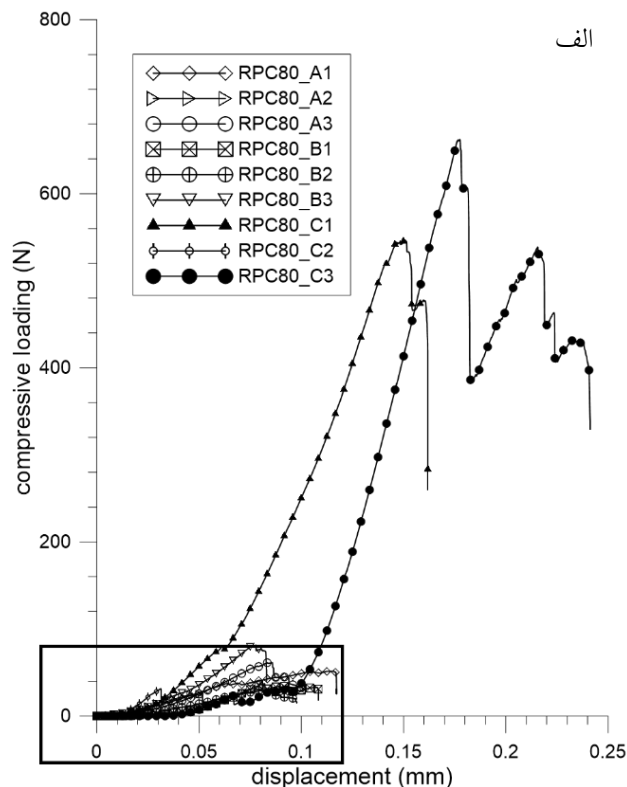
شکل ۳- الف) منحنی های نیروی فشاری - جابه جایی برای پایه های ماکرومتخلخل در اندازه حفره های مختلف، ب) بزرگنمایی قسمت
