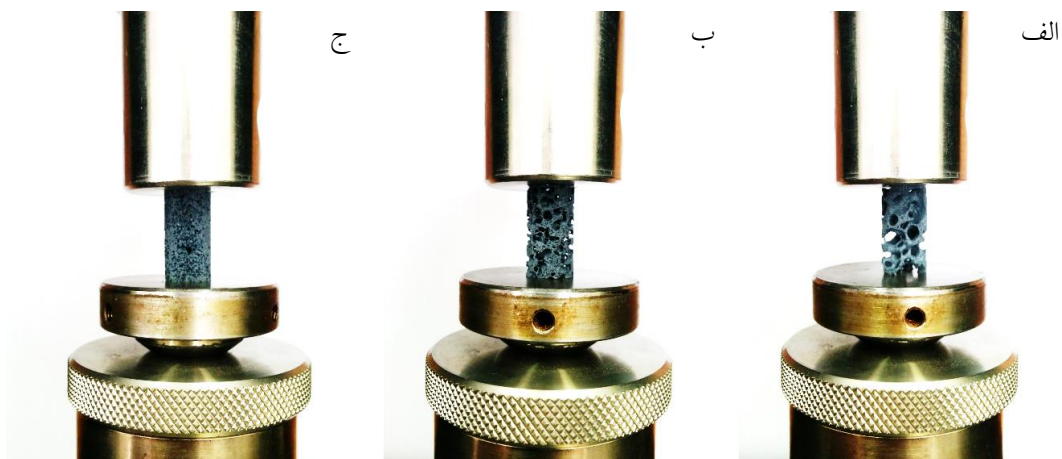
شکل ۱- نمونه‌های ماکرومتخلخل سرامیکی در اندازه حفره‌های مختلف و نحوه قرارگیری طی آزمون استحکام فشاری بر طبق استاندارد
