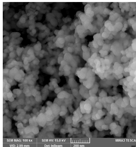
شکل ۱- تصویر میکروسکوپی الکترونی روبشی ثانویه ۵ (SEM-SE) از مورفولوژی پودر نانوزیرکونیای مورد استفاده
