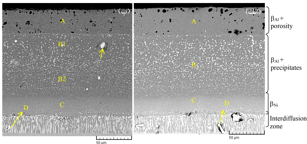
شکل ۳- نتایج مشخصه‌یابی و تصاویر میکروسکوپی الکترونی روبشی برگشتی از مقطع پوشش‌ها؛ الف) لایه آلومیناید بر لایه میانی نیکل و ب) لایه آلومیناید بر لایه میانی \text{Ni-ZrO}_2 ( \beta_{\text{Ni}} : فاز \text{NiAl} غنی از نیکل، \beta_{\text{Al}} : فاز \text{NiAl} غنی از آلومینیوم، پیکان به فازهای کاربیدی اشاره می‌کند).
