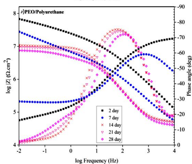
شکل ۱۰- نمودارهای باد-مدول و باد-فاز نمونه‌های: (الف) پوشش تک‌لایه اپوکسی، (ب) پوشش دولایه PEO/Epoxy، (ج) پوشش تک‌لایه FBE، (د) پوشش دولایه PEO/FBE، (ه) پوشش تک‌لایه پلی‌یورتان، (و) پوشش دولایه PEO/Polyurethane در طول چهار هفته غوطه‌وری در محلول ۳/۵ درصد وزنی NaCl (رنگی در نسخه الکترونیکی)
