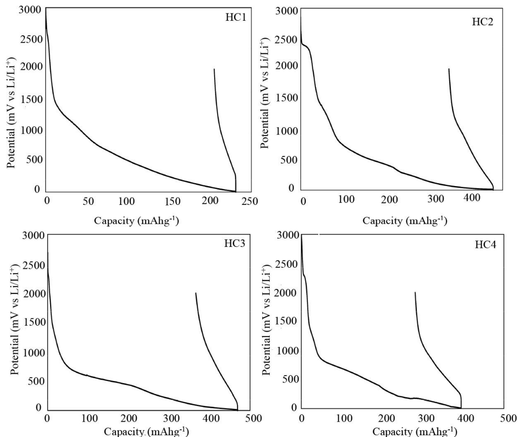
شکل ۷- نمودار چرخه اول شارژ و دشارژ مربوط به الکترودهای HC1، HC2، HC3 و HC4. نحوه انجام شارژ و دشارژ: شارژ تا ولتاژ ۱۰ میلی‌ولت با چگالی جریان ثابت ۱۰ میلی‌آمپر بر گرم، دشارژ تا ولتاژ ۲۰۰۰ میلی‌ولت با چگالی جریان ثابت ۱۰ میلی‌آمپر بر گرم
