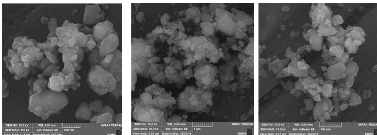
شکل ۹- تصاویر میکروسکوپی الکترونی گسیل میدانی نانوذرات سیلیکون تهیه شده با روش آسیاکاری مکانیکی با استفاده از آسیای سیاره‌ای پر انرژی با سرعت ۵۰۰ دور بر دقیقه و نسبت گلوله به پودر ۲۰ به ۱ به مدت ۲۴ ساعت، در بزرگنمایی‌های مختلف
