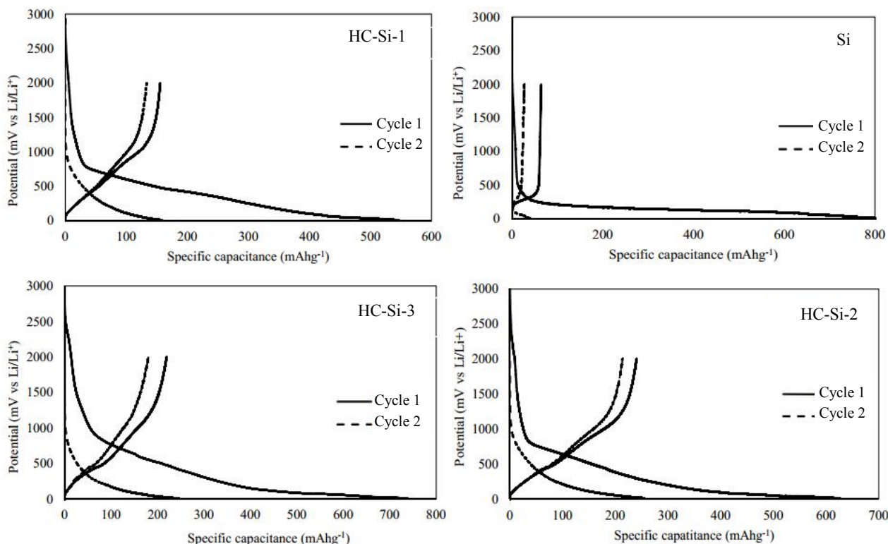
شکل ۱۱- چرخه اول و دوم شارژ و دشارژ کامل الکتروکود HC-Si-1، HC-Si-2، HC-Si-3 و Si
