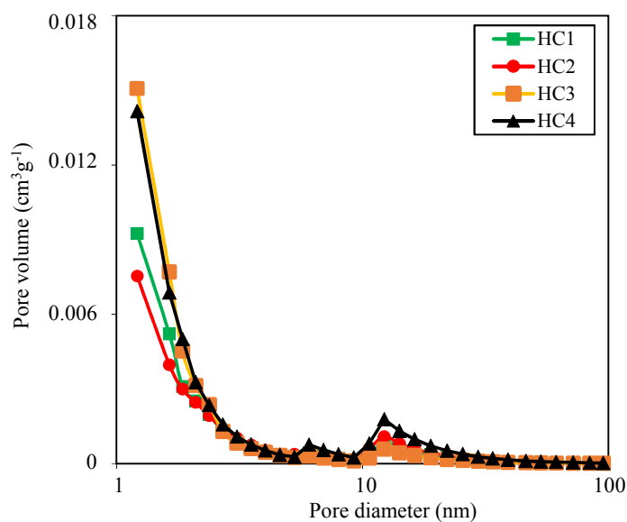
شکل ۶- نمودار BJH نمونه‌های کرین سخت
