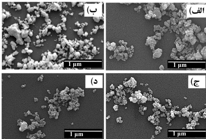
شکل ۹- تصاویر میکروسکوپی الکترونی روبشی از ذرات: (الف) ZrO 2 ، (ب) Z10S، (ج) Z20S، (د) Z30S و (هـ) نمودار اندازه متوسط ذرات
