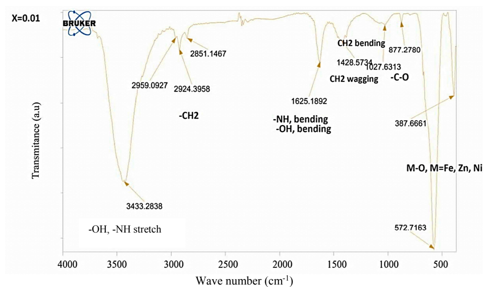
شکل ۷- طیف مادون قرمز با تبدیل فوریه نانوذرات \text{Ni}_{0.7}\text{Zn}_{0.3}\text{Nd}_x\text{Fe}_{2-x}\text{O}_4 به‌ازای x = 0.07 بعد از کلسینه کردن در دمای 750^\circ\text{C} درجه سانتی‌گراد
