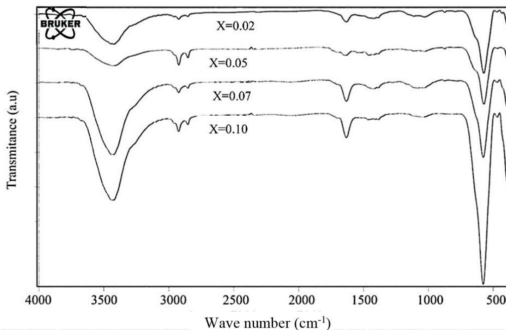
شکل ۸- طیف مادون قرمز با تبدیل فوریه نانوذرات \text{Ni}_{0.7}\text{Zn}_{0.3}\text{Nd}_x\text{Fe}_{2-x}\text{O}_4 به ازای x = 0.02, 0.05, 0.07, 0.10 بعد از کلسینه کردن در دمای 750^\circ\text{C} درجه سانتی گراد
