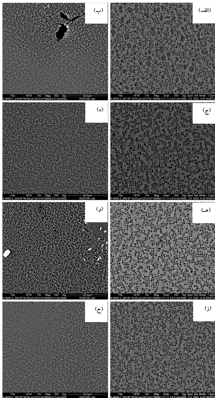
شکل ۱۰- تصاویر میکروسکوپی الکترونی روبشی از رسوبات ۷ در آلیاژهای مورد مطالعه: الف، ج، ه و ز) پس از عملیات حرارتی پیرسختی و ب، د، و و ه) پس از آزمون خزش نمونه‌های: الف و ب) SXM1، ج و د) SXM2، ه و و) SXM3 و ز و ح) SXM4
