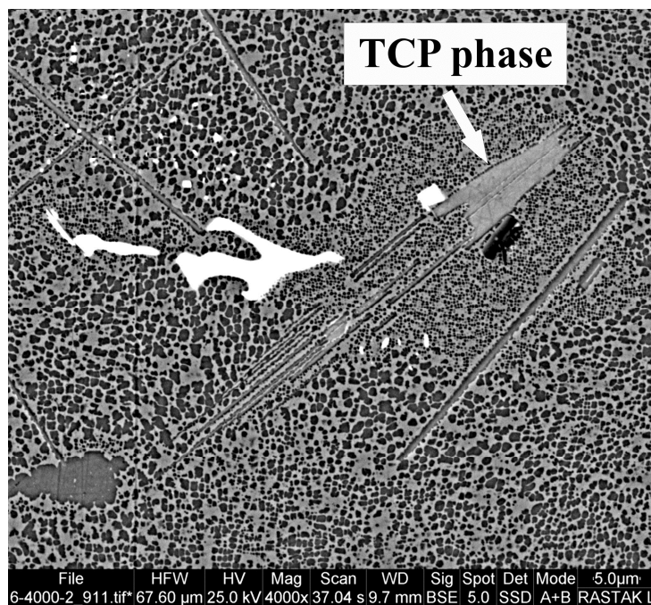
شکل ۶- تصویر میکروسکوپی الکترونی روبشی فاز TCP نوع \eta در ریزساختار آلیاژ SXM4 پس از عملیات پیرسختی
