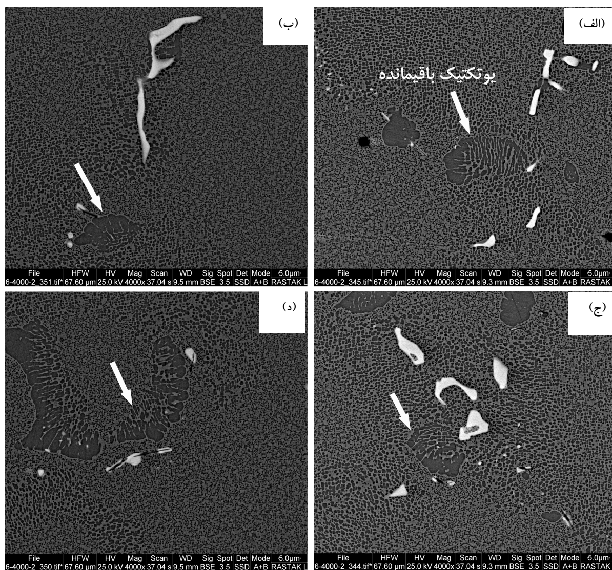
شکل ۴- یوتکتیک باقیمانده در ریزساختار نمونه‌های تک‌بلور پس از عملیات پیرسختی:
