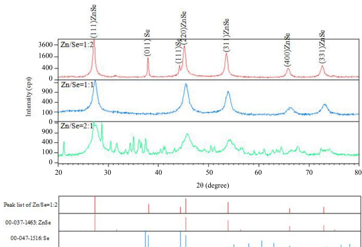
شکل ۱۱- الگوی پراش پرتو ایکس سلیکد روی در نسبت مولی مختلف \text{Zn}(\text{Ac})_2/\text{SeO}_2
