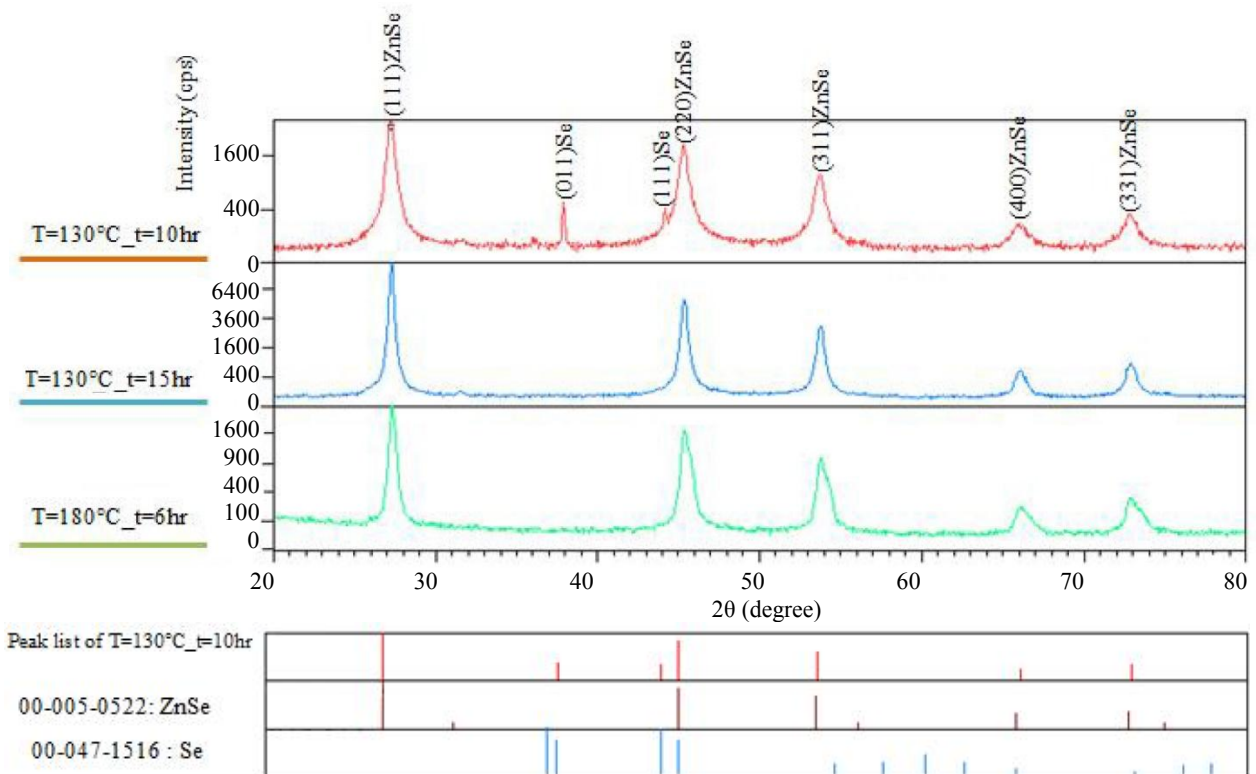
شکل ۷- الگوی پراش پرتو ایکس سلبید روی در زمان‌های مختلف سنتز در دمای ۱۳۰ درجه سانتی‌گراد
