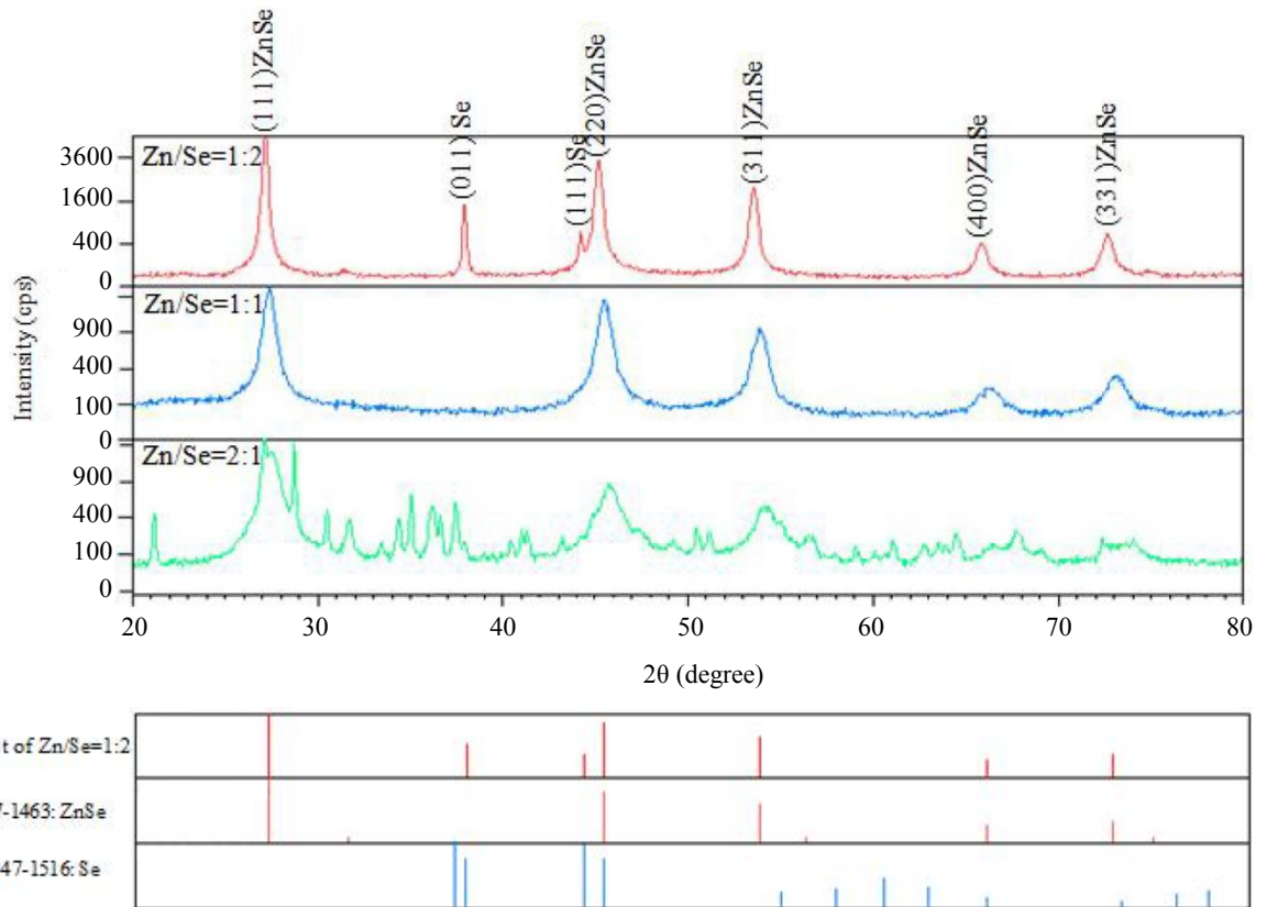
شکل ۱۱- الگوی پراش پرتو ایکس سلیکد روی در نسبت مولی مختلف Zn(Ac) 2 /SeO 2
