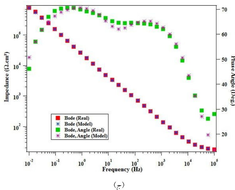
شکل ۱۸- نتایج انطباق نقاط به دست آمده از آزمون (منحنی‌های بد و بد- فاز) (Real) با نقاط حاصل از شبیه‌سازی توسط مدار الکتریکی (Model): الف) نمونه ۱، ب) نمونه ۲ و ج) نمونه ۳
