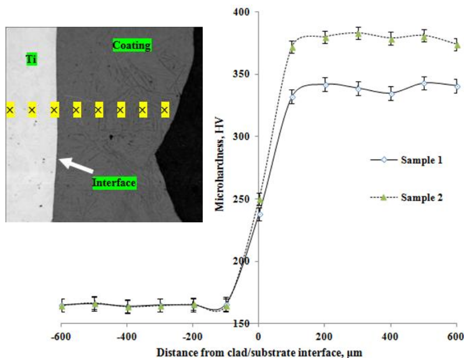
شکل ۱۰- تغییرات ریزسختی (ویکرز) پوشش‌های تهیه شده در یک پاس (Sample ۱) و دو پاس (Sample ۲) برحسب فاصله از فصل مشترک پوشش / زیرلایه (میکرومتر)
