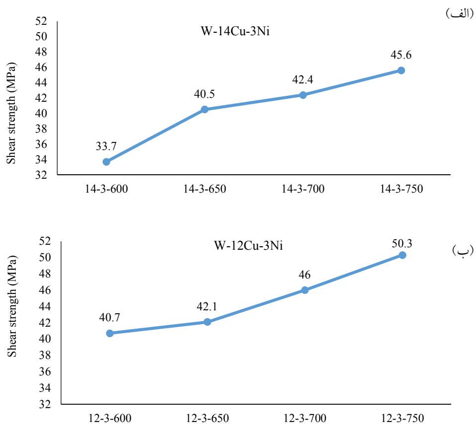
شکل ۵. نمودار تغییرات مقاومت برشی بعد از عملیات تف‌جوشی:
