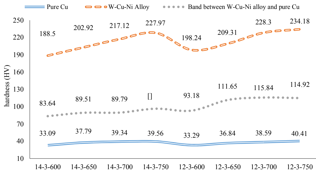
شکل ۴. سختی ویکرز کلیه نمونه‌های سیتتر شده (رنگی در نسخه الکترونیکی)
