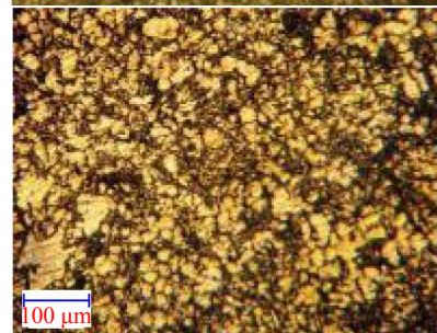
شکل ۶- تصاویر ریزساختار نمونه‌های ریخته‌گری با افزودن براده به سطح مذاب و کف بوت در دماهای مختلف (رنگی در نسخه الکترونیکی)
