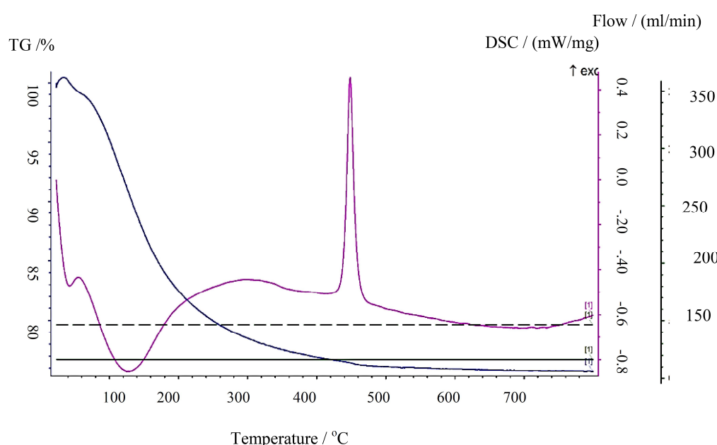
شکل ۸- نتایج آزمون توزین حرارتی و گرماسنجی افتراقی مربوط به نمونه C1
