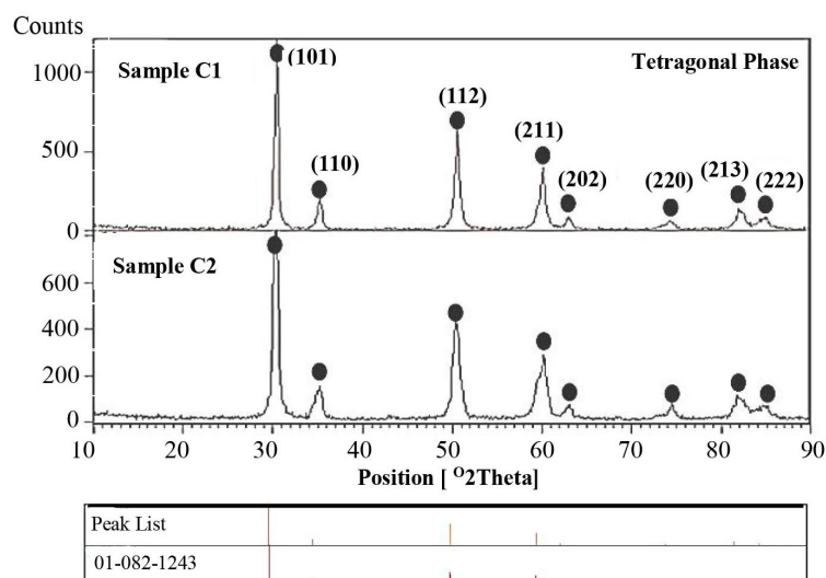
شکل ۱- الگوهای پراش پرتوی ایکس نمونه‌های YSZ سنتز شده به روش هم‌رسوبی نمونه‌های C1 و C2
