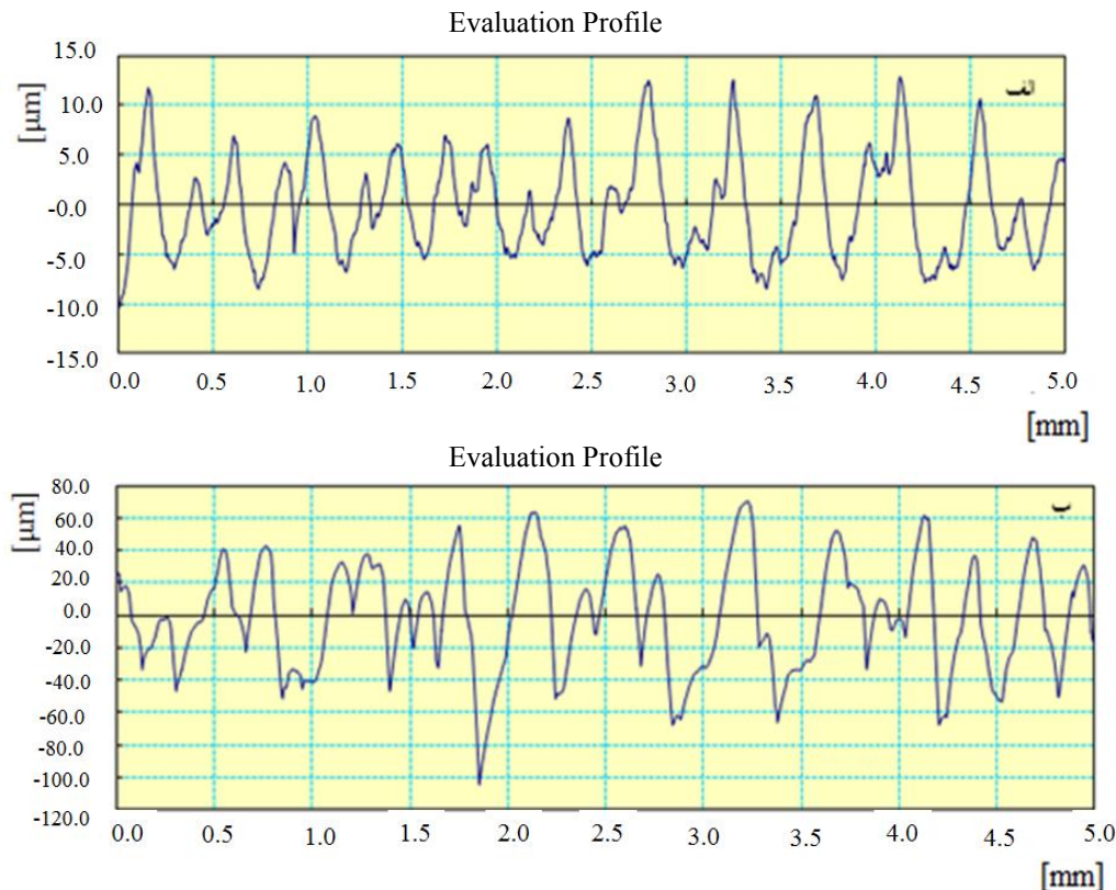
شکل ۹- منحنی زبری سنجی خطی از وجوه: الف) بالایی و ب) کناری یک نمونه
