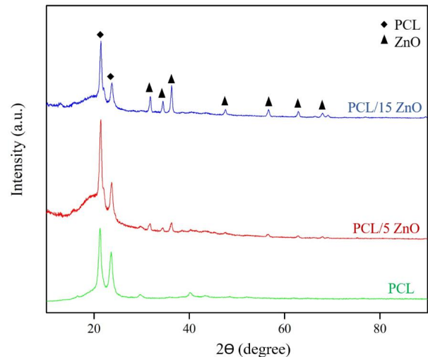
شکل ۱- الگوی پراش پرتو ایکس داربست‌های پلی‌کاپرولاکتون حاوی ۵، ۱۵ درصد وزنی نانوذرات اکسید روی.
