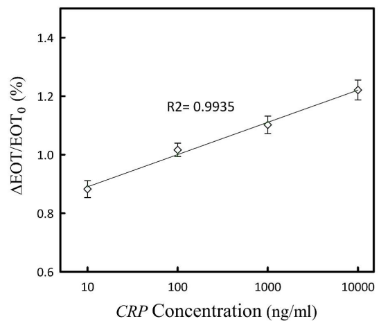
شکل ۵- پاسخ حسگر زیستی اصلاح شده با آپتامر پروتئین واکنش دهنده C به صورت نسبت تغییرات ضخامت نور مؤثر لایه برحسب غلظت‌های مختلف از پروتئین واکنش دهنده C.
