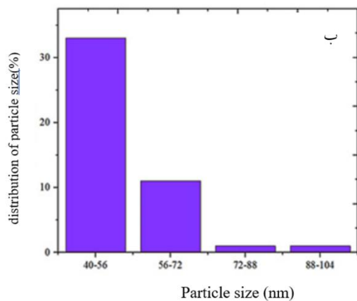
شکل ۴- هیستوگرام توزیع اندازه ذرات پودر: الف) آلفا آلومینا ب) گاما آلومینا، بعد از رسوب شیمیایی.
