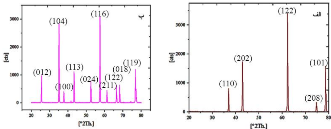
شکل ۲- الگوی پراش پرتو ایکس نمونه‌های: الف) آلفا آلومینا ب) گاما آلومینا، به همراه کمک تفجوش‌های اکسید منیزیم و اکسید لانتانوم، بعد از فرایند تفجوشی پلاسما جرقه‌ای.
