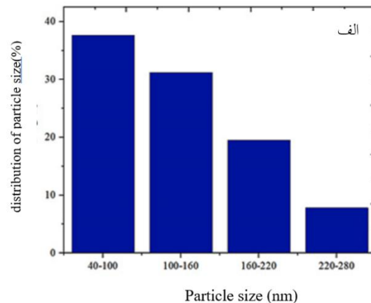
شکل ۴- هیستوگرام توزیع اندازه ذرات پودر: الف) آلفا آلومینا ب) گاما آلومینا، بعد از رسوب شیمیایی.
