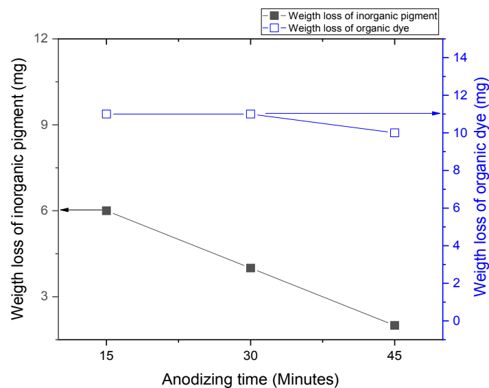
شکل ۵- نمودار تست سایش پوشش‌های آندایزینگ سیاه با ضخامت پوشش آندیک مختلف حاوی رنگدانه‌های معدنی (نمودار چپ) و آلی (نمودار راست).
